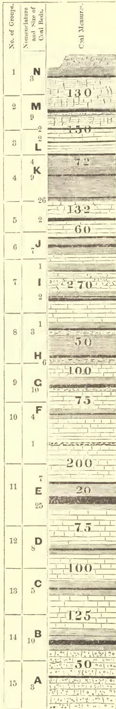
FIG. 1.—ANTHRACITE STRATA
